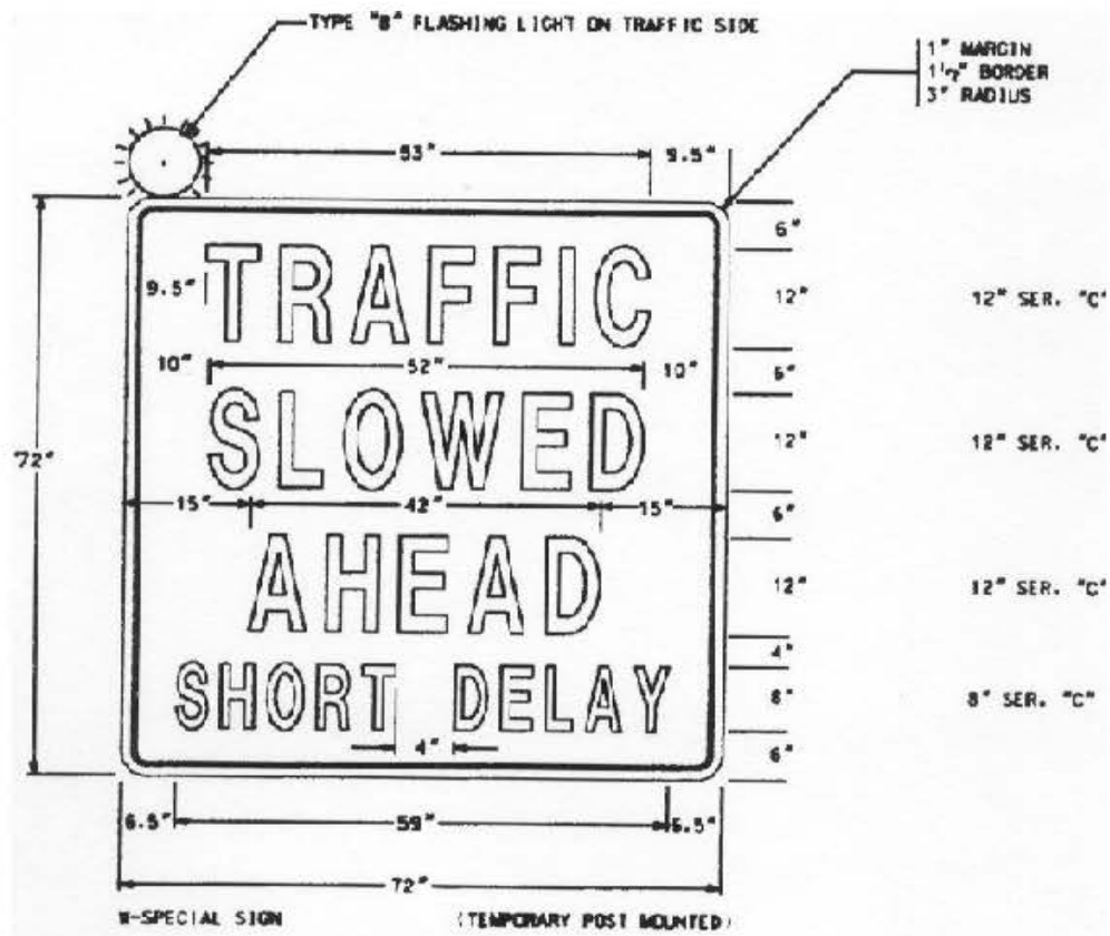
DETAIL 150-A
